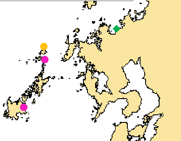
3月の漁船海難発生地点
