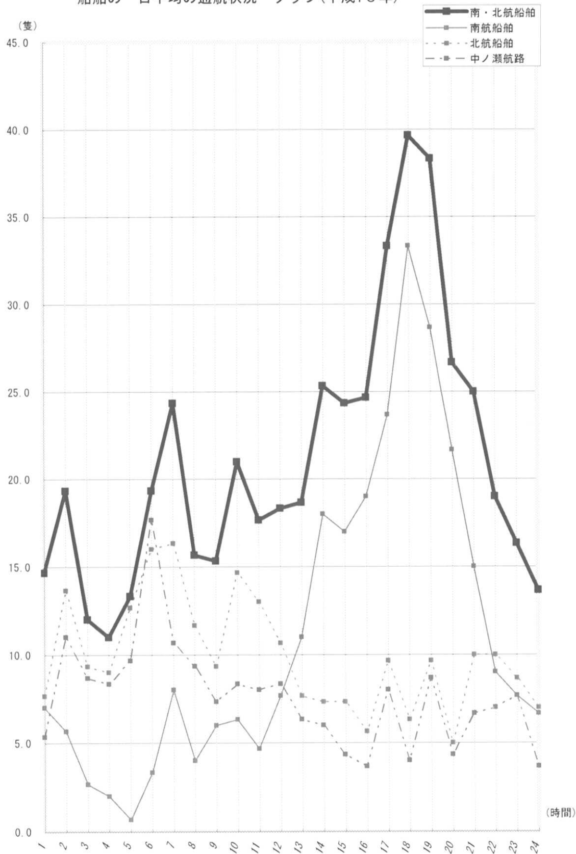
ハ. 浦賀水道航路及び中ノ瀬航路における時間別・方向別 船舶の一日平均の通航状況 グラフ(平成16年)
