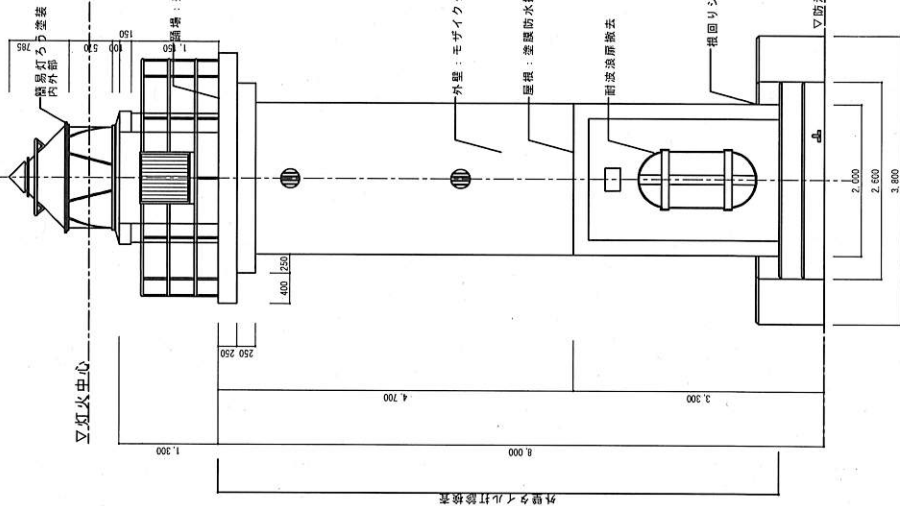
改修前正面図 1/50
