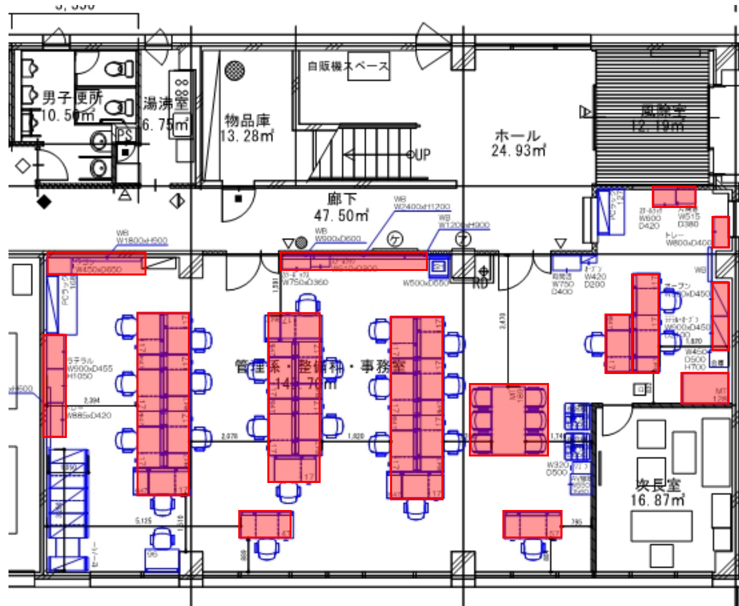
【別図1】 改修前 1 階執務室配置図
