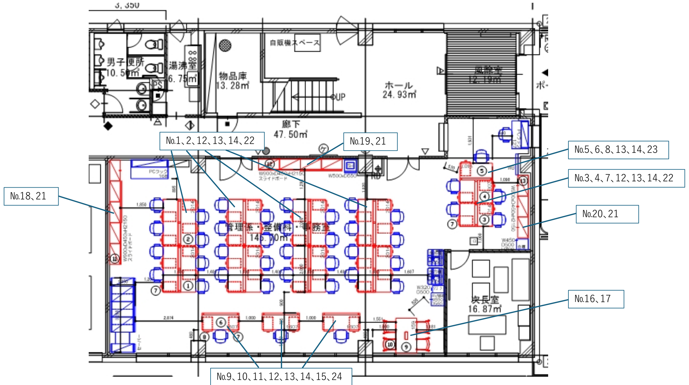
【別図2】 什器配置後 1 階執務室配置図
